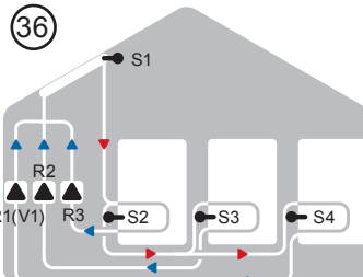
Solár se 3 zásobníky a 3 čerpadly
