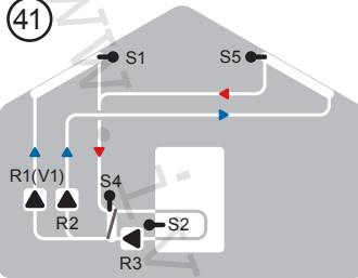
Solár se 2 kolektory, tepelným výměníkem, zásobníkem a 3 lerpady
