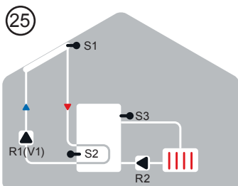
Solár s chlazením 3 (chlazení kolektoru)
