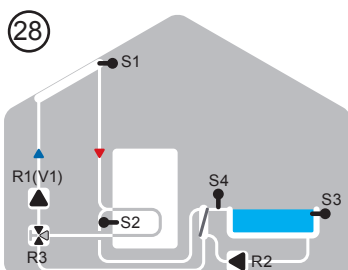
Solár s bazénem, zásobníkem, tepelným výmělníkem a ventilém
