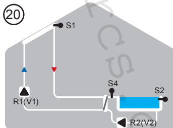
Solár s bazénem a tepelným výměníkem
