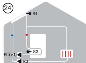
Solár s chlazením 2 (chlazení kolektorů)
