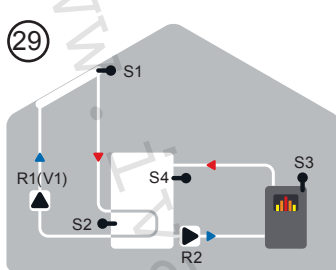
Solár se zásobníkem a kotlem na tuhá paliva a S4
