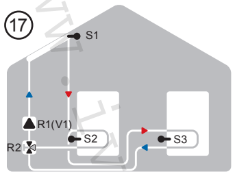
Solár se 2 zásobníky a přeplínacím ventilem
