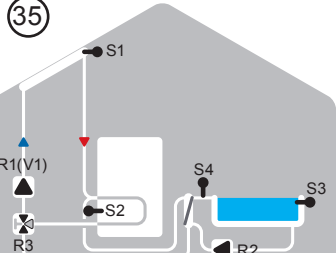
Solár s bazénem, zásobníkem, tepelným výmělníkem a ventilém
