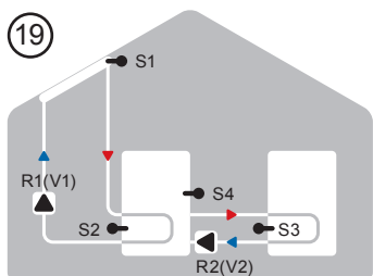
Solár s přenosem mezi zásobníky
