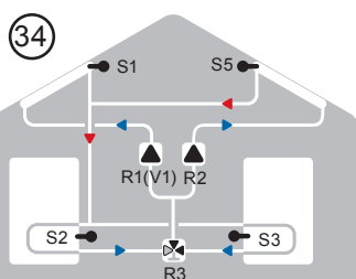
Solár s 2 kolektory, 2 zásobníky a 2 čerpadly
