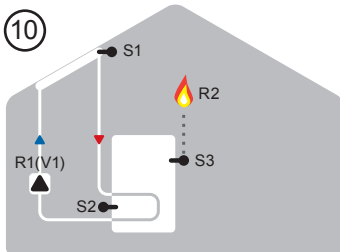
Solár s termostatem (přídativně vytápění)
