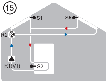
Solár s 2 kolektory a plepínacím ventilem
