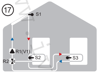
Solár se 2 zásobníky a plepínacím ventilem
