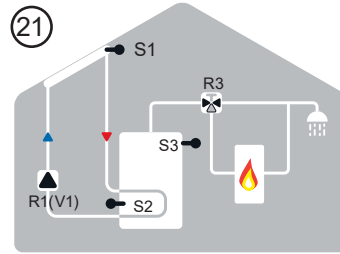
Solár s termostatem a plepínacím ventilem
