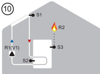
Solár s termostatem (přídavné vytápění)
